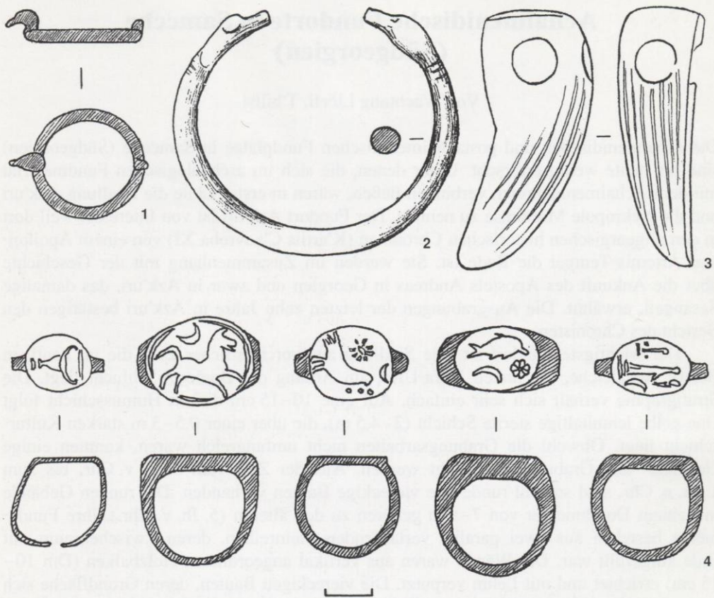
Abb. 1. 1 Azk'uri. Bronzering (1. Jh. n. Chr.); 2 Msetamse. Bronzearmreif (5. Jh. v. Chr.); 3 Azk'uri. Knochenring aus Eberzahn (5.-4. Jh. v. Chr.); 4 Azk'uri. Bronzesiegelringe (5.-4. Jh. v. Chr.).
